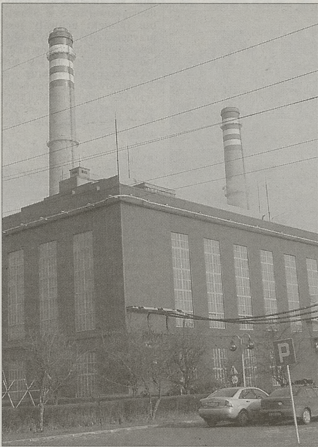
W hali maszynowni i kotłowni zamontowano dźwiękochłonne okna znacznie ograniczające wydobywający się hałas
