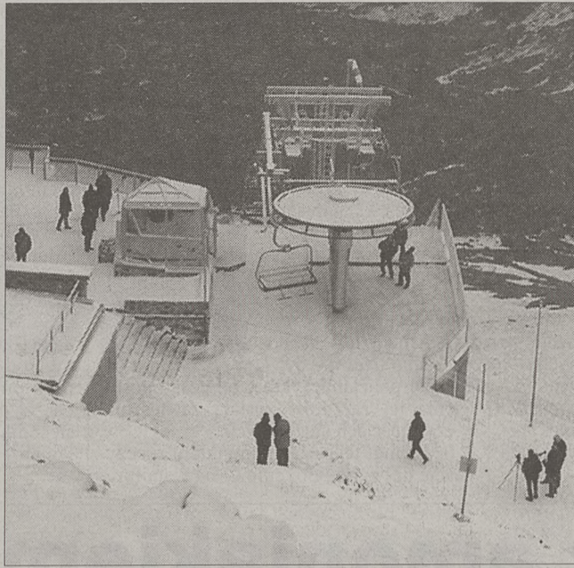
Nowa górna stacja kolei krzesełkowej w Kotle Gąsienicowym
