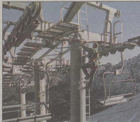
Zakończyła się, trwająca 202 dni, budowa nowoczesnego wyciągu krzeselkowego na Hali Gąsienicowej. 4-osobowy wyciąg o długości ponad 1200 m może przewieźć 2400 osób na godz. Do 15 grudnia trwały prace rozruchowe.
