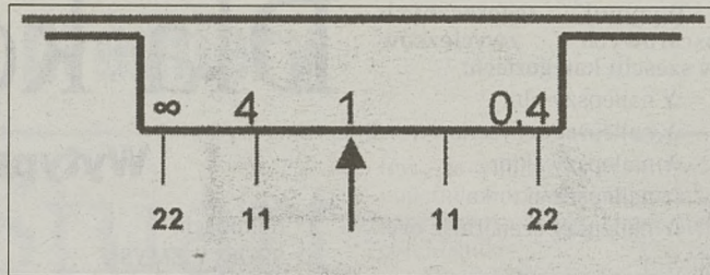
Odległość hiperfokalna 1 m: głębia ostrości przy przysłonie 22 sięga od 0,4 m do nieskończoności (obiektyw 20 mm).
