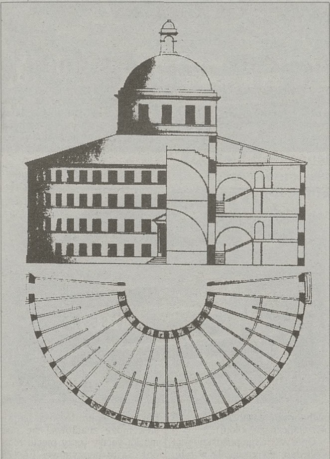
Projekt wszystkowidza; rzut poprzeczny i pionowy
