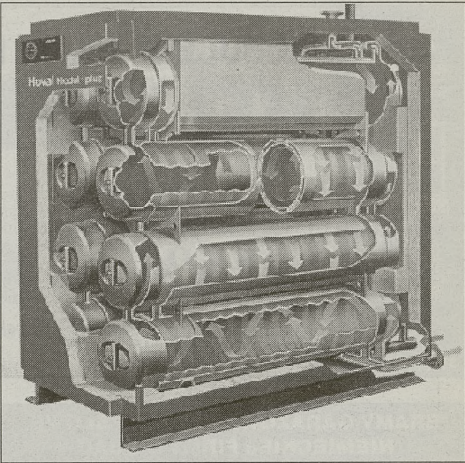
Podgrzewacze o budowie modułowej
