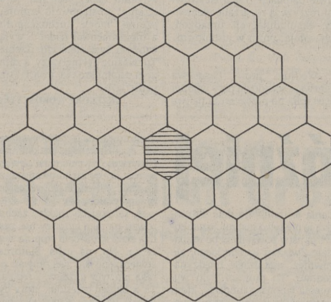
Schematyczny wygląd zwierciadła teleskopu Keck I
