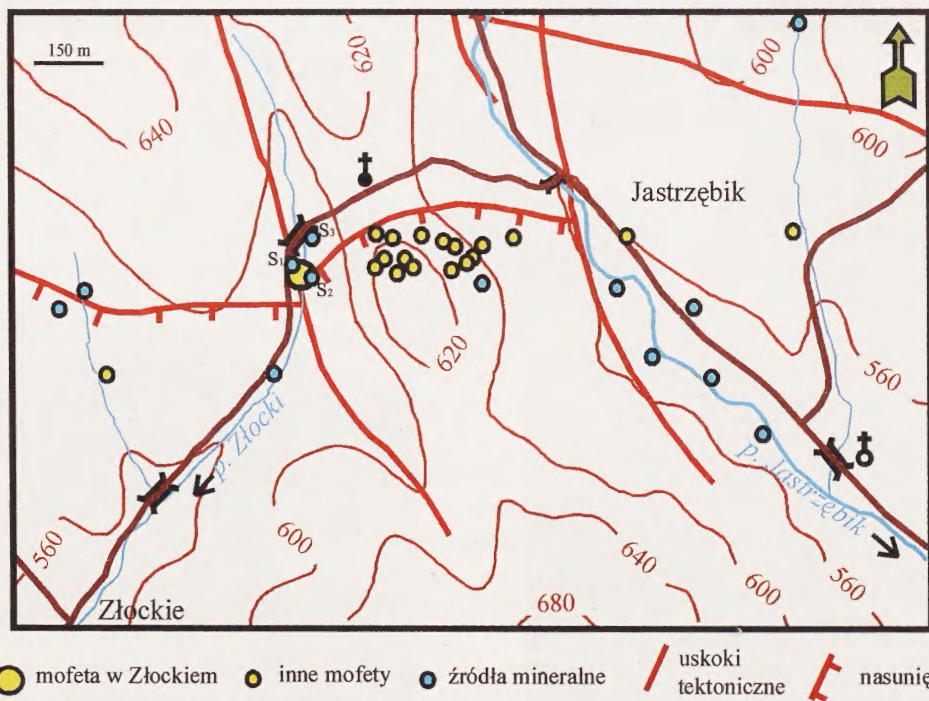
3. Szkic sytuacyjno-tektoniczny rejonu Złockiego - Jastrzębika
