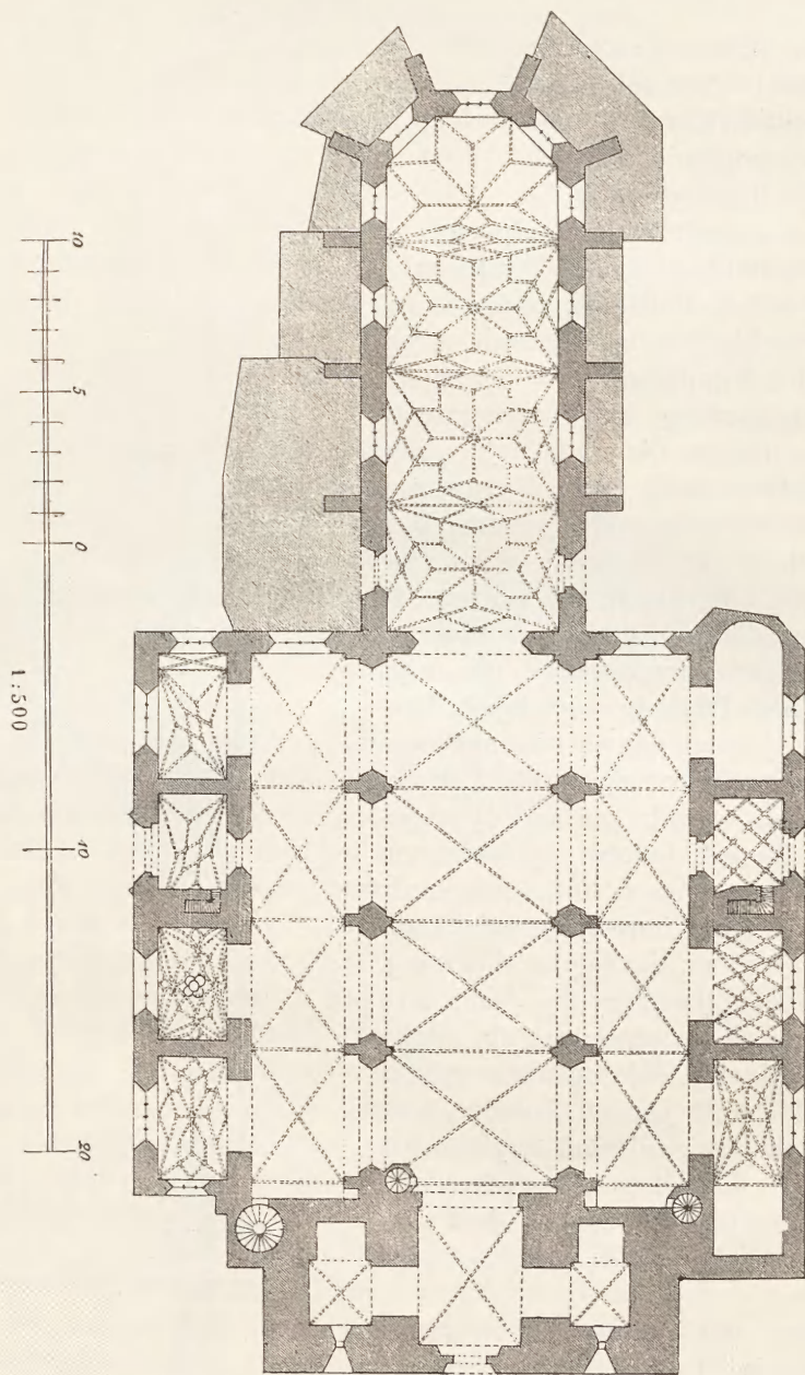
Rys. 6. Rzut kościoła N. P. Maryi w Krakowie (według Essenweina).
