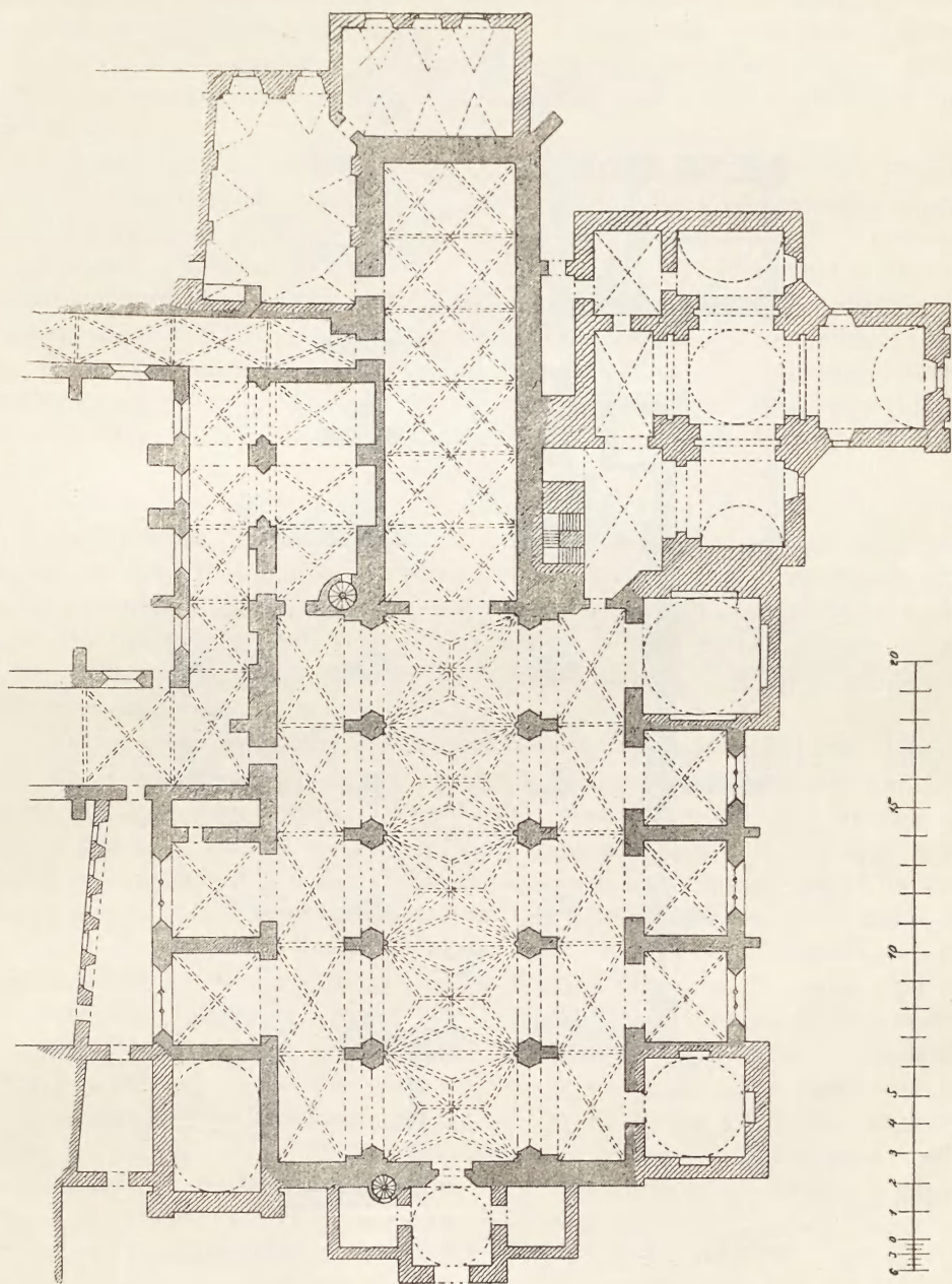
Rys. 8. Rzut kościoła Dominikanów w Krakowie (według Essenweina).
