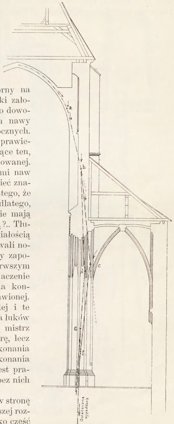
Rys. 5 Z kościoła św. Katarzyny w Krakowie. Linia ciśnięć
