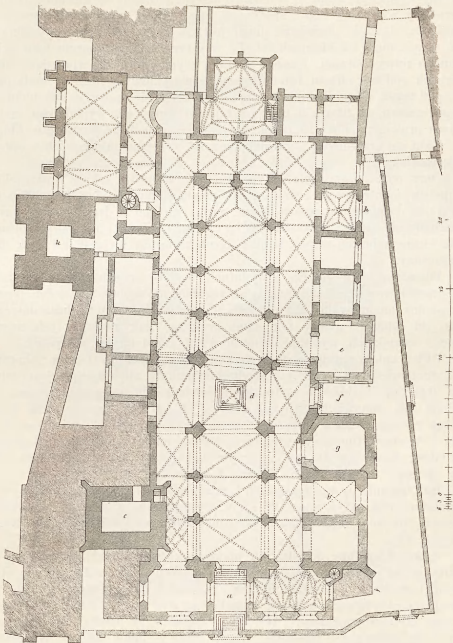
Rys. 7. Rzut kościoła katedralnego na Wawelu (według Essenweina).
