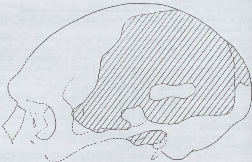
Rekonstrukcja czaszki z Ganoviec (wg Vlček 1950)
