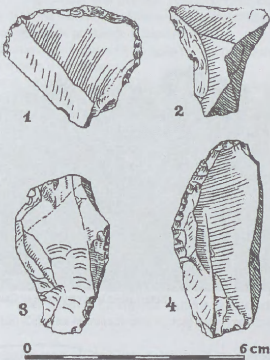
Horka-Ondrej. Wyroby kamienne (wg Łożek, Prošek 1957)
