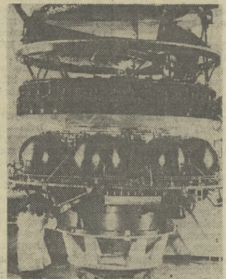
W tym roku Japonia umieści na orbicie swego pierwszego satelity telekomunikacyjnego „JCSAT”. Górna część (dysk anteny) będzie stacjonarna i skierowana ku Ziemi, by zapewnić całonocową, nieprzerwaną łączność. Część dolna (m. in. zespół napędowy) będzie zastąpiła cylindryczną powłoką pokrytą płytkami — ogniwami słonecznymi, które dostarczać będą przetworzoną energię słoneczną. Część ta będzie obracać się jak żyroskop, dla zapewnienia statyczności satelity.
