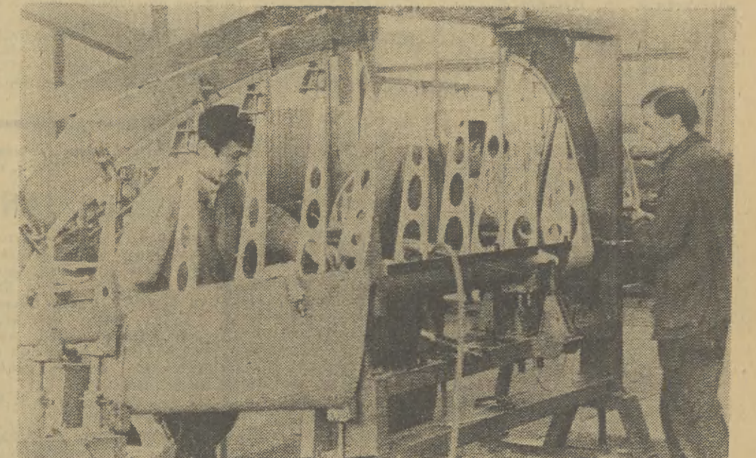
Na zdjęciu: produkcja usterzeń do samolotów AN-2 w gospodarstwie Kombinatu „Igloopol” w Puszkowie. Fot. WACŁAW KŁAG
