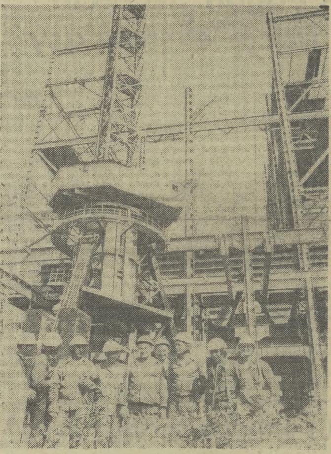
Zmontowano już finalny element ostatniego słupa konstrukcji budynku głównego dla „spiećki” elektrowni Kozienice. Chłopcy z Energomontażu — ludzie-ptaki — wisząc w specjalnych koszach na dużej wysokości zmontowali około 4500 ton konstrukcji. Trzeba do takich operacji gorącego serca, złotych rąk, stalowych nerwów i znajomości ekwilibrystyki. CAF-Stan
