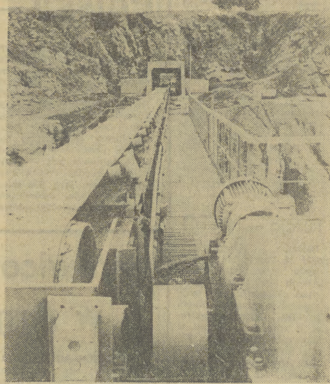
Postępująco największe w świecie złoża rudy niklu, Kuba znajduje się w czołwie producentów tego cennego surowca. Na zdjęciu: w prowincji Oriente przy wydobyciu rudy niklu zainstalowano nowoczesne urządzenia transportowe produkcji radzieckiej. CAF — Pr. Latina
