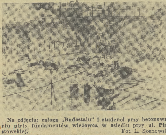
Na zdjęciu: załoga „Budostalu” i studenci przy betonowaniu płyty fundamentów wieżowca w osiedlu przy ul. Piastowskiej. Fot. L. Sosnowski
