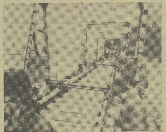
Na trasie Szczecin—Swinoujście trwa modernizacja linii kolejowej. Układają się m. in. tory na łukach o większym promieniu — pozwoli to na większą szybkość pociągów, przewożących głównie węgiel do portu w Swinoujściu. N/Z: układanie torów. CAF — Undro — telefoto
