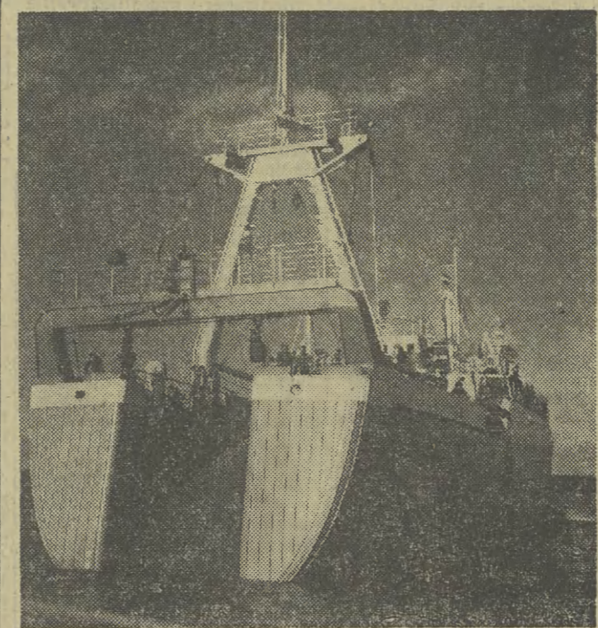
Jednostki tego typu co widać na zdjęciu trawler-pretwornia „Peniks” łowiła w ciągu roku 6 do 7 tys. ton ryb. Całe nasze rybołówstwo na najlepszym roku przedwojennym odловиło 23 tys. ton ryb morskich. CAF — fot. Ukłejewski
