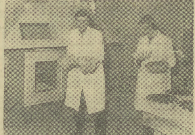
Pracownica Zakładu Anna Maziarz przenosi pokryte teftonem foremki pod lampy, gdzie będą leżakować tak długo, aż wyschną. Następnie przeniesione zostaną do pieca, i wypalane w temp. 400 stopni. Na drugim zdjęciu inż. Wiesław Korcała wyjmuje gotowe formy. Fot. W. Klag
