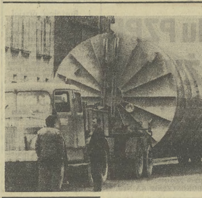
Blisko milion kuflów piwa wyprodukować będzie można w tej gigantycznej kadzi o wymiarach 4,5 x 22,5 m, transportowanej od producenta w Karl-Marx-Stadt do browaru w Stornburgu.
