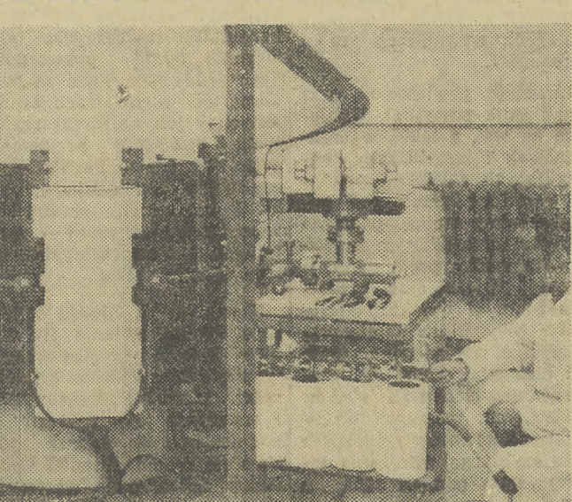
W Polkowicach trwa — rozpoczęły w pierwszej dekadzie bm. — rozruch pierwszego akceleratora cząstek Beta. Betatron będzie dokonywał analiz i oznaczał zawartość miedzi w rudzie oraz w produktach flotacji. Zastępuje 20 laborantów pracujących metodami tradycyjnymi. Czynność pomiaru trwa 10 minut, a wynik gotowy jest w ciągu 2 godzin. Od stycznia 1972 betatron w Polkowicach wyeliminuje całkowicie stosowane dotychczas metody chemiczne, pomoże również w dalszych badaniach geologicznych. Na zdjęciu: przy rozruchu betatronu mgr Mikołaj Potocki i mgr inż. Kazimierz Komisaruk.
