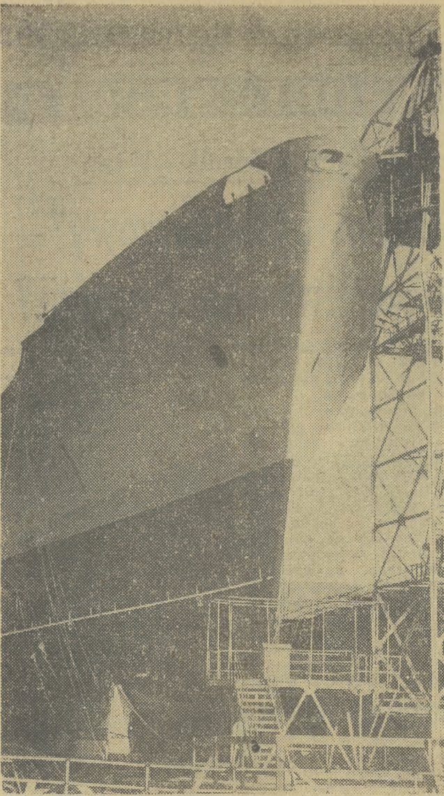
22 bm. w Stoczni Szczecińskiej Im. Adolfa Warskiego zawodowany został nowego typu 10-tysięcznik przeznaczony dla PLO. Nosi on nazwę „Mieszko I”. Na zdjęciu: M/S „Mieszko I” na pochylu „Odra” w Stoczni Szczecińskiej. CAF — Wezzer
