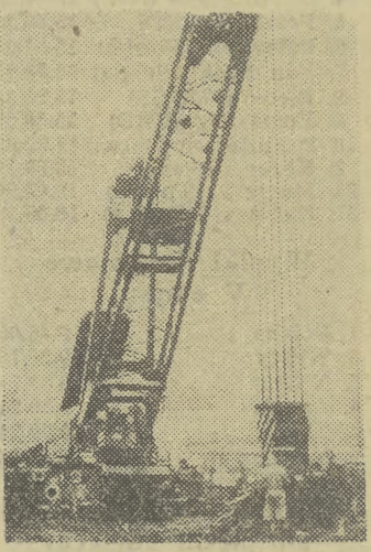
Próba jednego z dwóch nowych dźwigów kolejowych na dziedzińcu fabryki Smeral w Brnie (Czechosłowacja). Dźwigi umocowane są na obrzygniach podwoziach, ważących 120 i 156 ton. Sam dźwieg ma 28 metrów wysokości i może unieść do 125.000 kg. CAF — CTK
