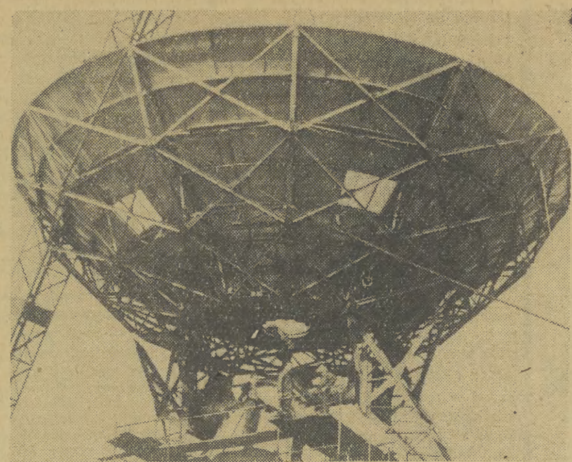
TAK OTO WYGLĄDA ANTENA NOWEGO RADIOTELESKOPU MONTOWANEGO NA FORCIE SKALA POD KRAKOWEM (Do artykułu: obok) fot. Jerzy Kreiner
