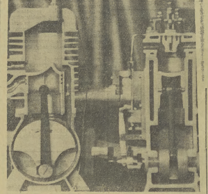
Model silnika dwutaktowego — górnosuwowego i silnika diesla.
