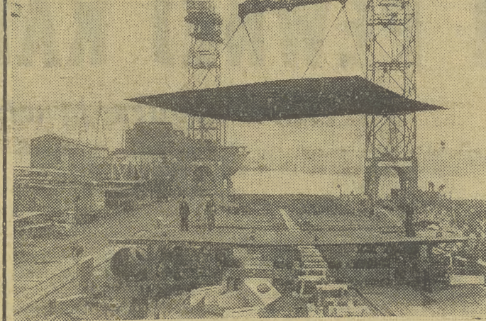
W stocznim im. Adolfa Warskiego w Szczecinie położono stępkę pod nowy typ statku B-516 (drobnicoowiec o nośności 8200 DWT), którego konstrukcję opracował mgr inż. Eugeniusz Haćski. Na zdjęciu: moment kładzenia stępki. CAF — fot. Wecezer
