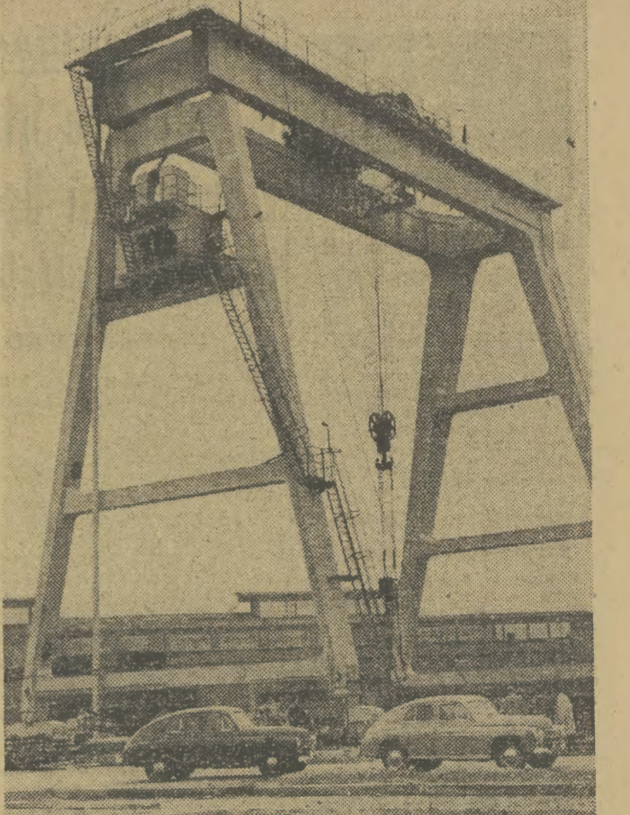
W Stoczni Szczecińskiej im. A. Warskiego oddano do użytku największą w polskim przemyśle okrętowym suwnicę bramową, która będzie mogła przemieścić i ustawiać na pochylni gotowe elementy kadłubów statków o wadze do 100 ton. Suwnica została wykonana przez stoczniowców według dokumentacji „Prozamec”. Na zdjęciu: suwnica bramowa na pochylni „Wulkan”. CAF — fot. Szczołowski
