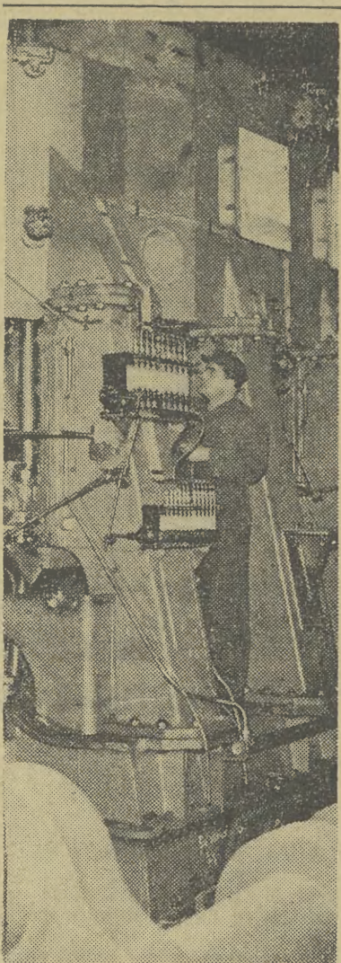
Zakłady H. Cegielskiego w Poznaniu produkują m. in. maszyny okrętowe typu TR-800 o mocy 800 KM, przeznaczone do trawlerów rybackich.
