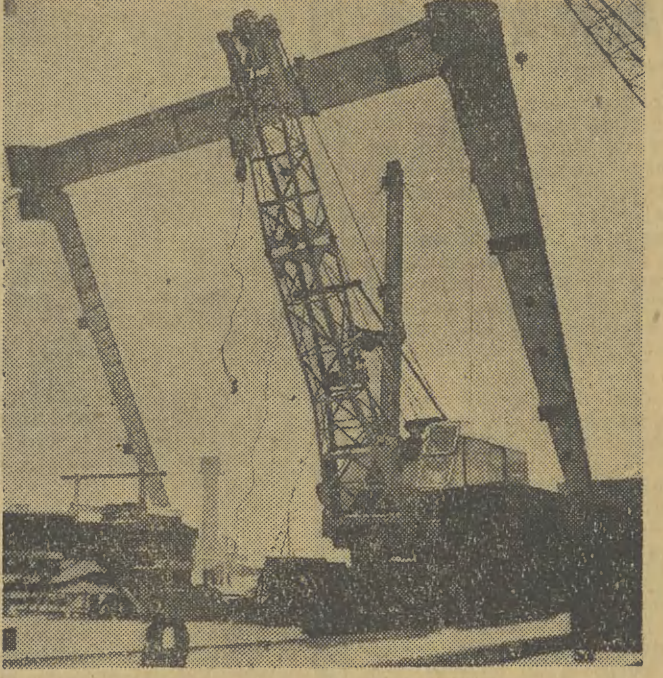
W Stoczni Szczecińskiej Im. Adolfa Warskiego postawiono pierwszą część słupów bramyowej o szerokości 25 metrów, która w dużym stopniu umożliwi skrócenie czasu montażu kadłubów dziesięciotysięczników. Na zdjęciu: Ustawienie słupów bramyowej.
