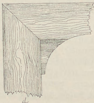
Ryc. 101 a—e. Zastrzały.
