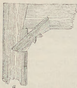
Zastrzał czyli es najprostszy z szopy Króla z pod Gu- bałówki.
