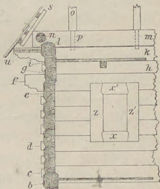
Rys. 3. Pionowe przecięcie części domu w podłuż.
