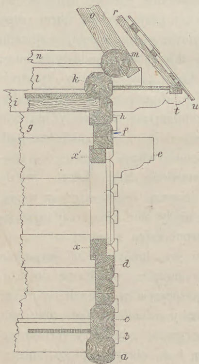
Rys. 2. Pionowe przecięcie części domu w poprzek.
