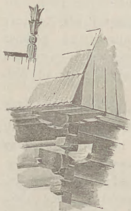
Rys. 6. Węgiel z rysiami i pazdur u góry (podług rys. p. W. Witkiewicza).
