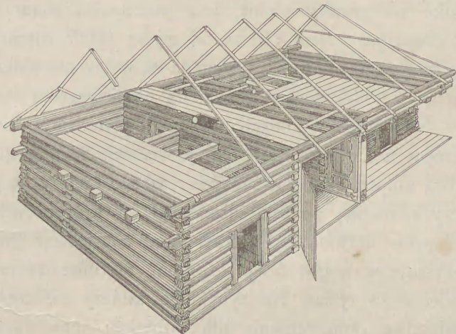
Rys. 20. Pokazujący budowę szopy.
