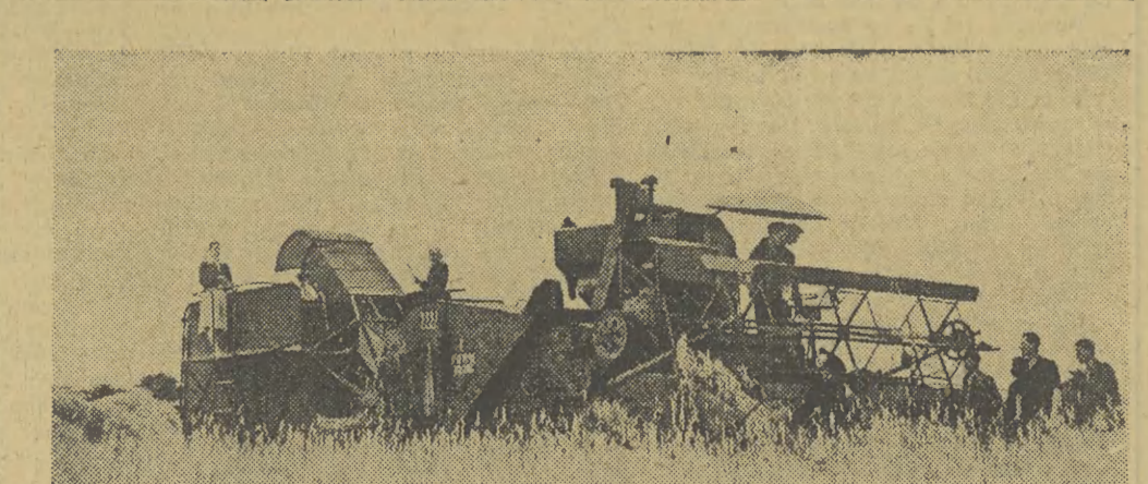
Dzięki pracy kombajnu spółdzielni produkcyjnej „Jedność” w Janiszewsku pow. Tczew zakończyła sprząć żyta. Na zdjęciu: Kombajn węgierski AC-400 z POM Rudno na polach spółdzielni
