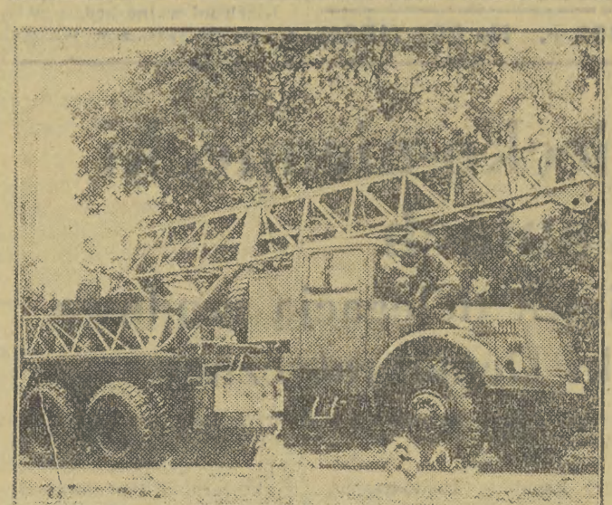
Załoga Fabryki Budowy Maszyn Im. Swiermy w Pradze. Wysozczany (Czechosłowacja) wykonuje na zamówienie Chińskiej Republiki Ludowej obrotowe dźwigi samochodowe. Dźwigi te umieszczone są na platformie Tatra 111 i podnoszą ciężary ok. 4 ton. Na zdjęciu: gotowy dźwig. Fot. CAF
