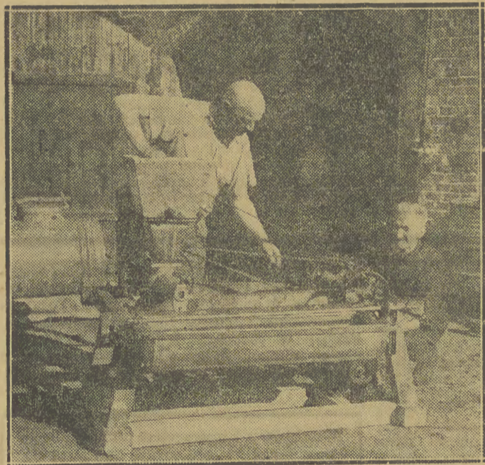
Dyrektor zespołu PGR Bloniz w pow. kutnowskim, Stanisław Leźnicki skonstruował wygniatarkę do owoców i warzyw, pozwalającą na oddzielenie pestek od miąższu bez uszkodzenia samego nasienia. Wydajność wygniatarki obliczona jest na 360 kg na godzinę i daje 93 proc. oszczędności robocizny. Na zdjęciu: dyrektor Leźnicki sprawdza działanie wygniatarki. OAF — fot. Szarhara
