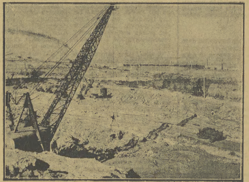
Praca przy wykopie pod fundamenty gmachu Elektrowni Kujbyszewskiej.
