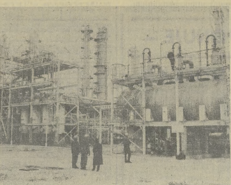
Budowa wytwórni PCW w Zakładach Azotowych „Włocławek” to czołowa inwestycja ostatnich lat, wznoszona przez zagranicznych wykonawców. Po zakończeniu budowy wszystkich obiektów będzie się tu wytwarzać rocznie około 200 tys. ton PCW. Na zdj.: widok na instalacje do produkcji chlorku winylu.
