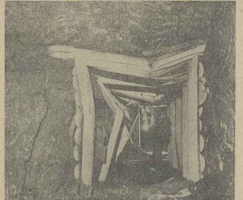
To zdjęcie ilustruje niszczącą działalność górotworu na wielkich wyrobiskach. Pod wpływem ciśnienia skał solidne drewniane obudowy łamią się jak zapalki.
