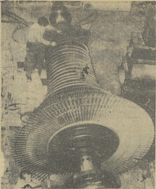
W elektrowni w Skawinie „kuracji odmładzającej” wymaga 6 turbozespołów. Fot. MICHAŁ KASZOWSKI
