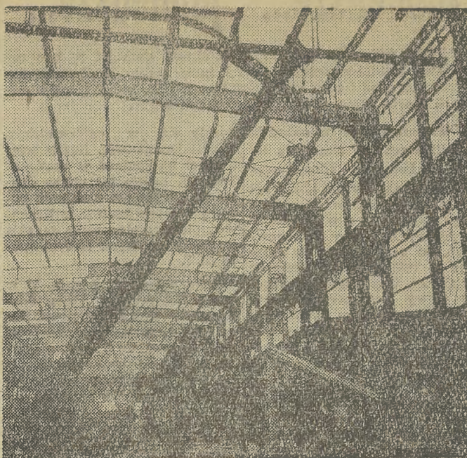
Rosną nowe obiekty walcowni zimnej blach karoseryjnych Kombinatu Huta im. Lenina. Fot. MICHAŁ KASZOWSKI
