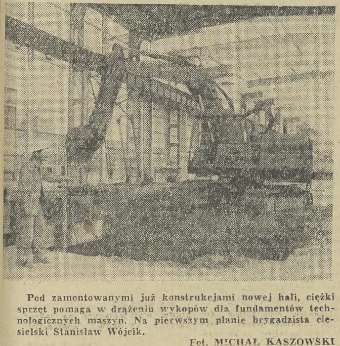
Pod zamontowanymi już konstrukcjami nowej hali, ciężki sprzęt pomaga w drażeniu wykopów dla fundamentów technologicznych maszyn. Na pierwszym planie brygadziści cieśli Stanisław Wójcik. Fot. MICHAŁ KASZOWSKI
