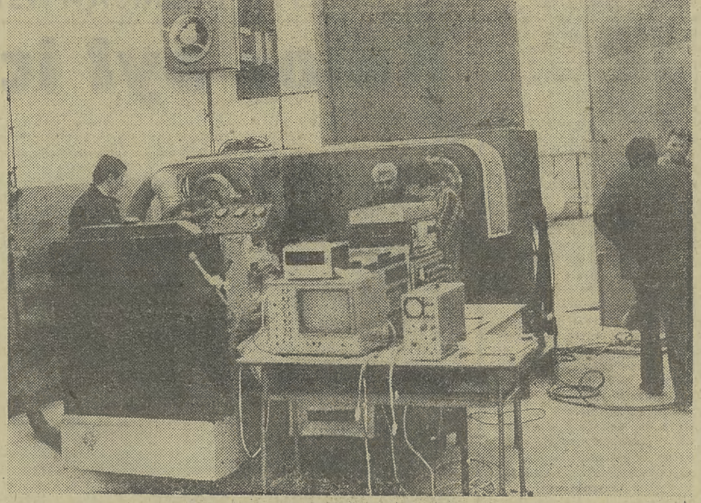
Na naszym zdjęciu badanie wykonanych w Instytucie Pojazdów Samochodowych i Silników Spalinowych PK, części prototypu ciągnika gąsienicowego (zbudowanego głównie na zespołach polskich) z urządzeniami do automatycznego i półautomatycznego spawania rurociągów. Wprowadzenie ciągnika do produkcji pozwoli na obniżenie kosztów importu o około 50 procent.
