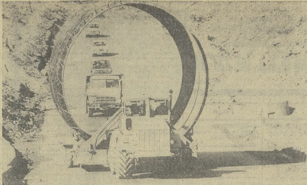
Transport urządzeń do montażu kolejnych bloków energetycznych Nureckiej Elektrowni Wodnej (ZSRR).
