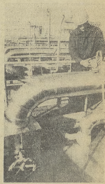
W Smolnie (dawnej Baszni) — doświadczalnie-produkcyjnej kopalni siarki, prowadzi się badania nad zastosowaniem technologii wydobycia siarki metodą podziemnego wytopu w tutejszych warunkach geologicznych. Metoda ta z powodzeniem stosowana jest od lat w kopalniach w Grzybowie i Jezioroku, jednak w odmiennych niż lubawowskie warunkach geologicznych. Pierwsze tony siarki z doświadczalnej kopalni w Smolnie już wydobyto. Na zdjęciu: Edward Mazurkiewicz reguluje dopływ wody do pola górnego. CAF — Lokaj
