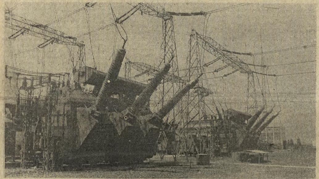
Transformatory na stacji wysokich napięć zbudowane według projektów krakowskich autorów. Fot. M. LOZIŃSKI
