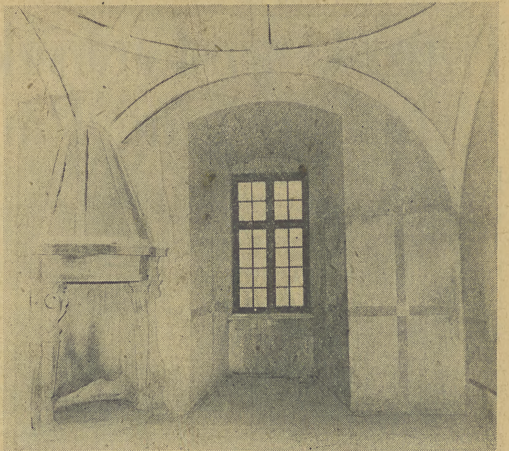
Oto fragment akustycznej sali na zamku w Wiśniczu. Po prawej stronie narożnik — słowa najciszej tu nawet szepcane, są doskonale słyszalne w drugim, przeciwległym narożniku i odwrotnie. Piękny kominek, to element dekoracyjny, niezwiązany z efektami akustycznymi. Fot. JADWIGA RUBIŚ
