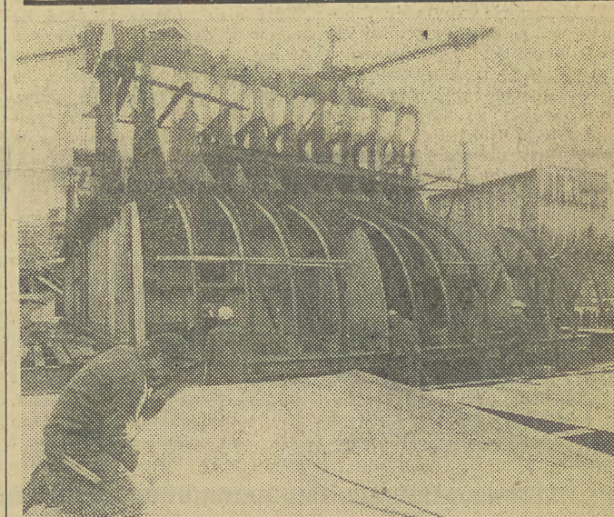
W Stoczni Szczecińskiej im. A. Warskiego położono stępkę pod pierwszy polski prom pasażersko-samochodowy, budowany na zlecenie Polskich Linii Oceanicznych. N/z: budowa pierwszego promu pasażersko-samochodowego. CAF — Undro
