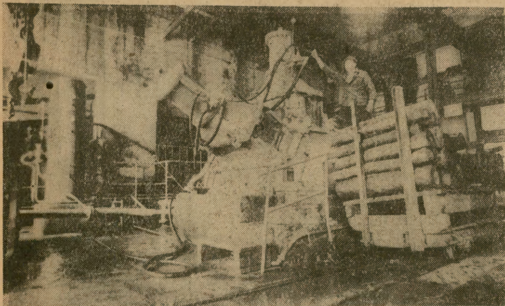
Sclerak w Białym Dunajcu w całej swojej okazałości. W nim rozpoczyna się pierwszy, a i najważniejszy etap przetworzenia drewna w tekturę.
