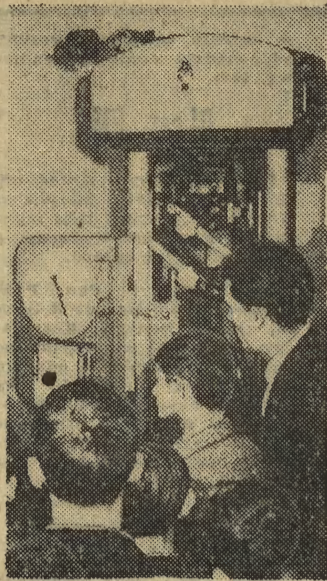
Uniwersalna maszyna do badania metali, pozwala na przeprowadzenie doświadczeń z zakresu rozrywania, ściskania, wybozczenia i zginania metali. Na zdjęciu: uczniowie w czasie przeprowadzania doświadczenia na rozrywanie
