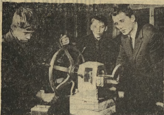
Na tej zaś maszynie pod kierunkiem mgr inż. J. Bielaszki uczniowie badają metodą Eriksena twardość blach. Doświadczenie to pozwoli im na lepsze zrozumienie zmian zachodzących w metalu, zaobserwowanych w czasie pracy w warsztatach, w których przez 3 dni w tygodniu zapoznają się praktycznie z zawodem.
