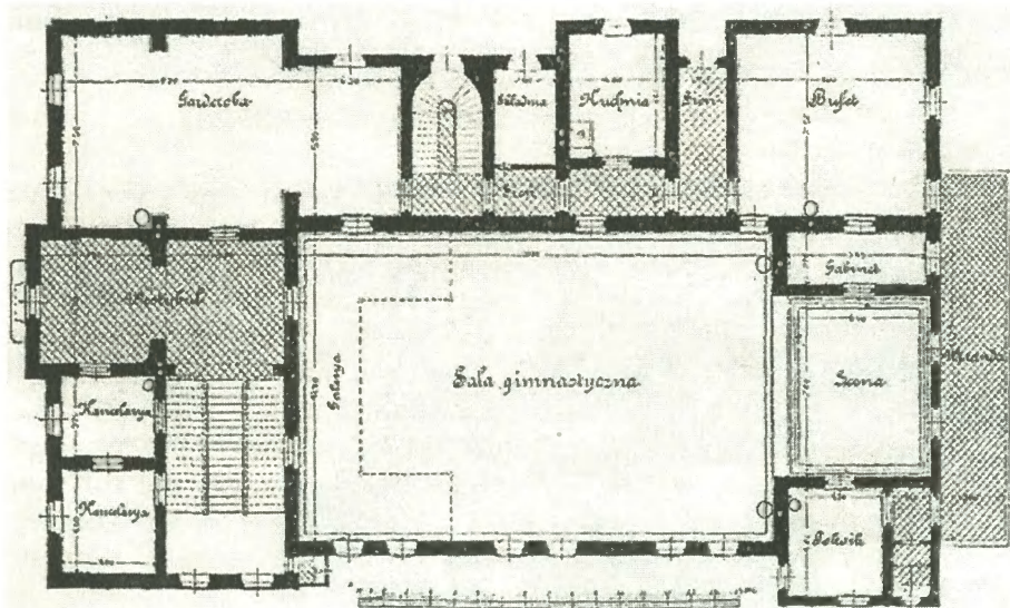
Plan pomieszczeń wnętrza budynku TG „Sokół” w Rzeszowie
