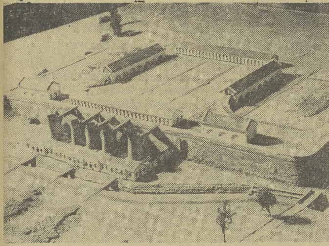
Rekonstrukcja wielkiej huty w Bobrzy dokonana przez pracowników Instytutu Urbanistyki i Architektury w Warszawie pod kierunkiem prof. dr W. Ostrowskiego. Budowę huty rozpoczął w 1818 r. Stanisław Staszic, a przerwano ją po wybuchu powstania listopadowego. Na zdjęciu widać na lewo zaporę i zbiornik wodny, 5 wielkich pieców, u góry estakada, plac fabryczny i hale magazynowe. Do dziś zachowały się części murów oporowych, fundamenty wielkich pieców i ruiny hal otaczających plac fabryczny. (Do art. obok.)
